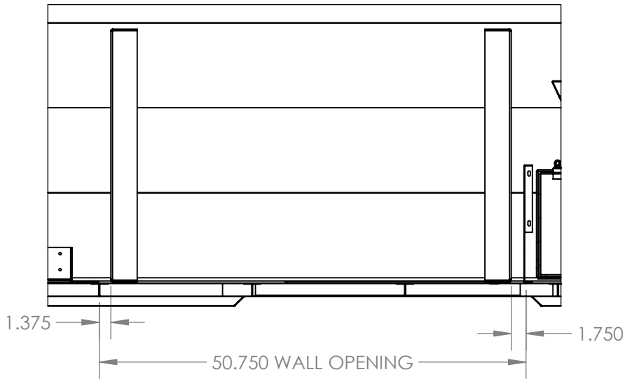
SECTION A-A SCALE 1 : 16
